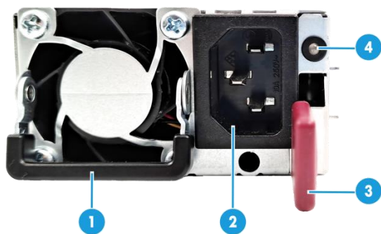
图9 DSP 电源模块前面板示意图
