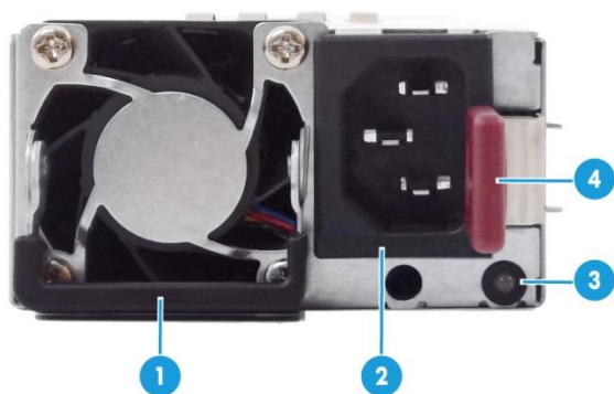
图8 PSR 电源模块前面板示意图
