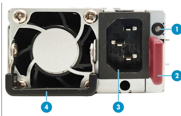
图7 GW 电源模块前面板示意图
