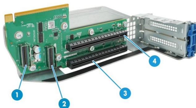
图11 RC-2LP-SlimSAS-2U Riser 卡
